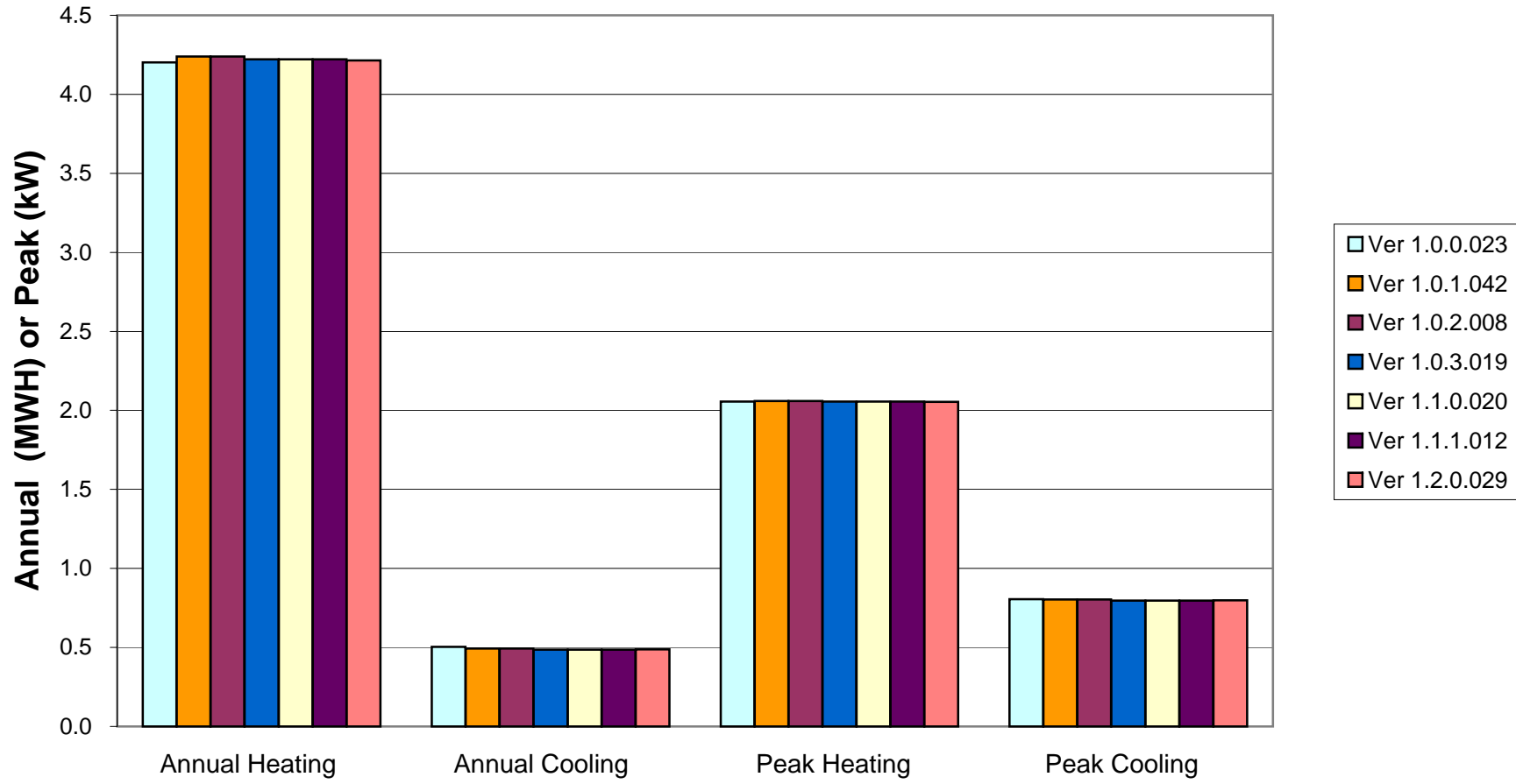
BESTEST Case 195
